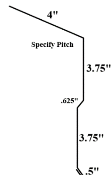
Step Eave (2X8)
