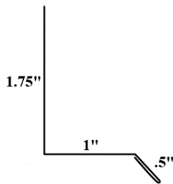
Step Eave (2X6)
