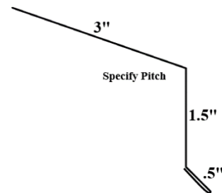
Step Eave (2X8)
